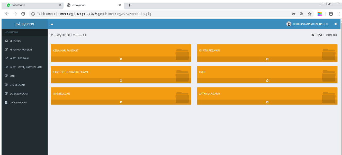
Halaman Utama
