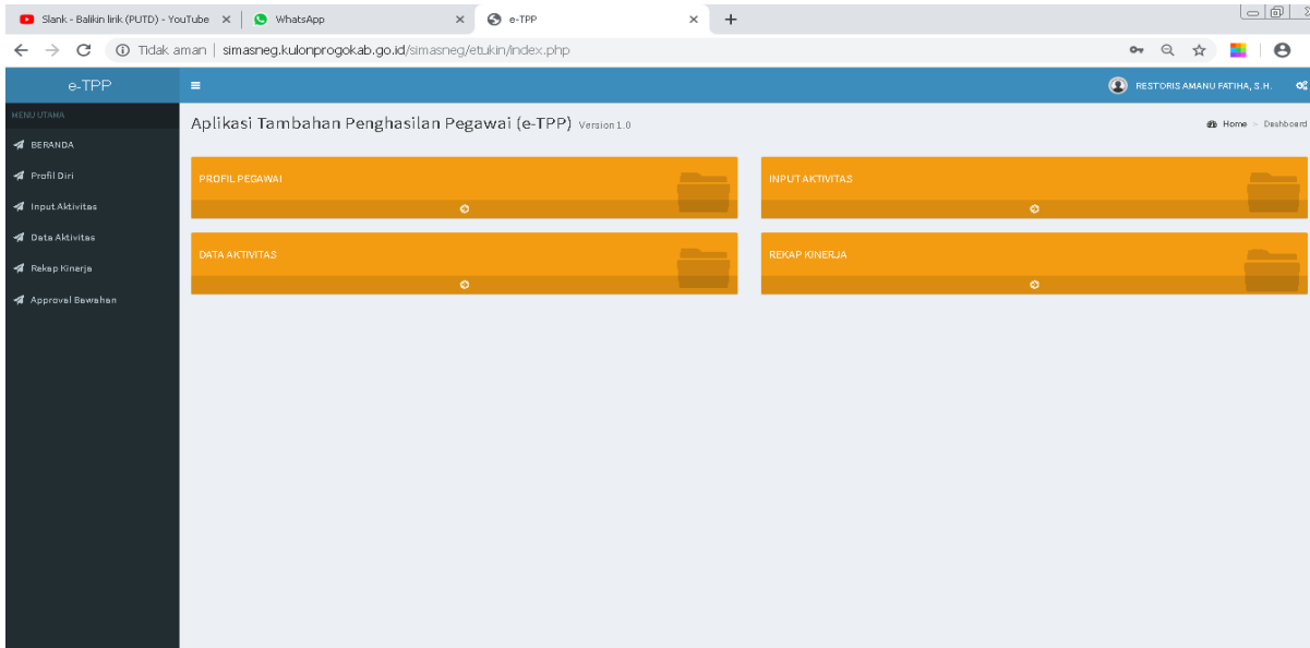
Halaman Beranda
