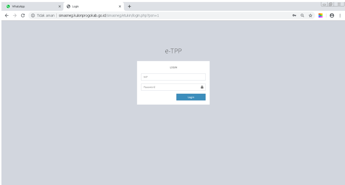
Halaman Login
