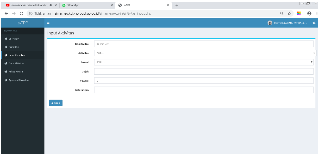
Input Aktivitas
