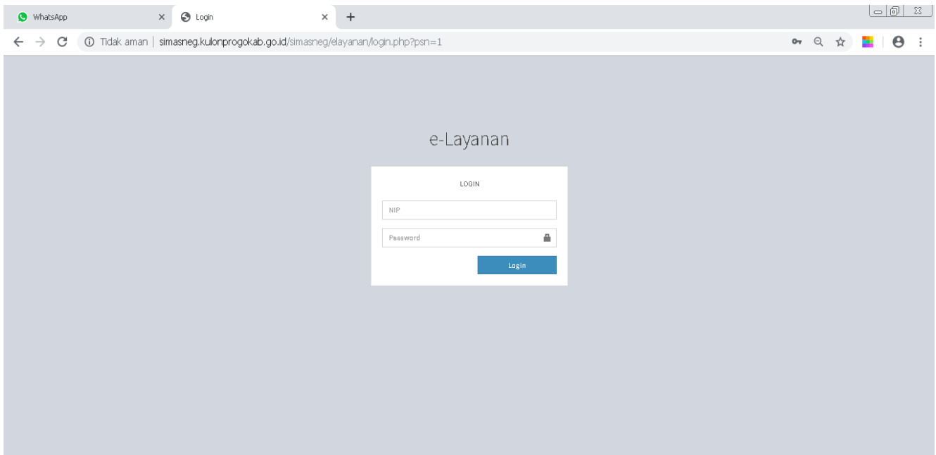
Halaman Login
