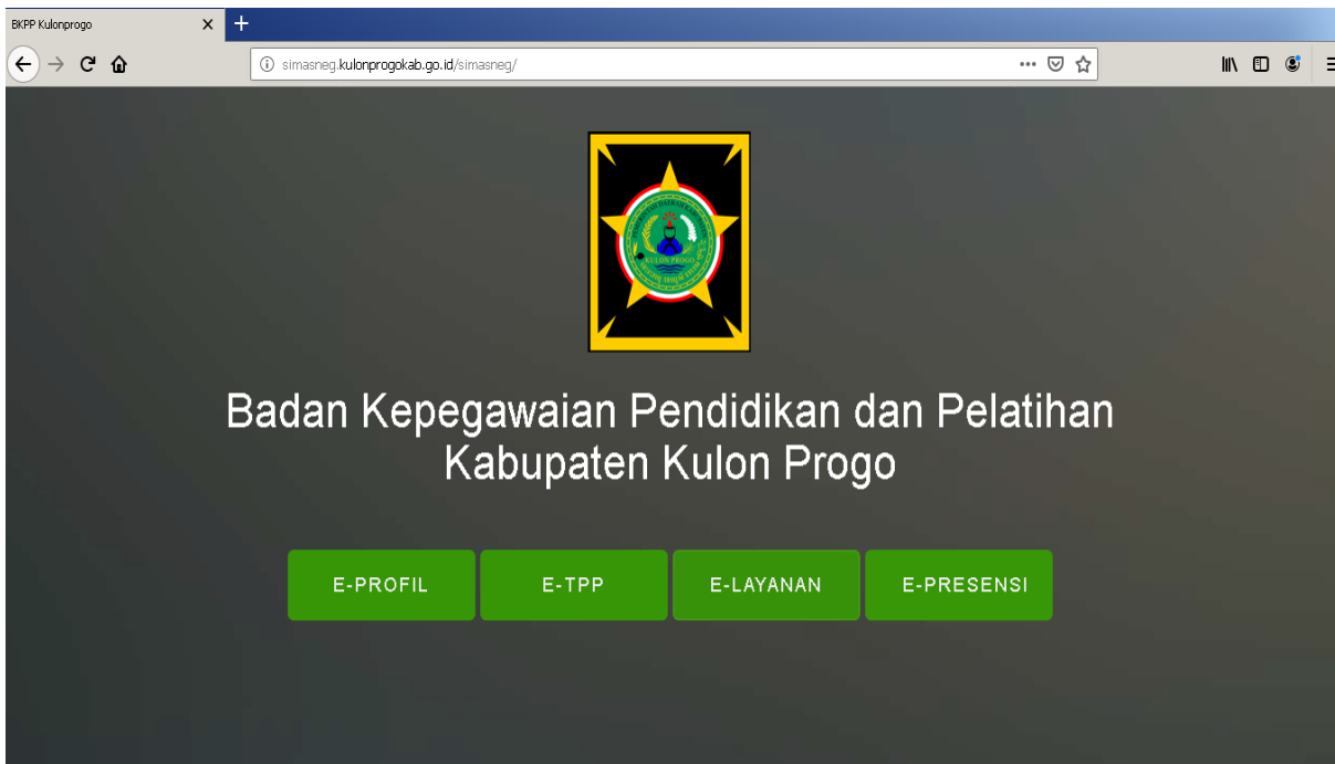
Halaman Utama
