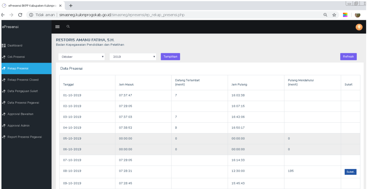
Rekap Presensi
